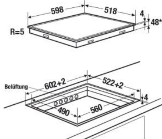
KI 6800.0 SR, GR flächenbündig
