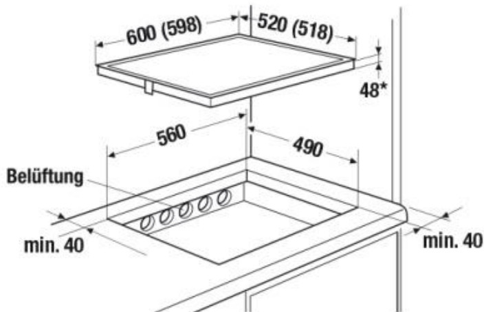
KI 6800.0 SF, (GR, SR) Aufsatz
